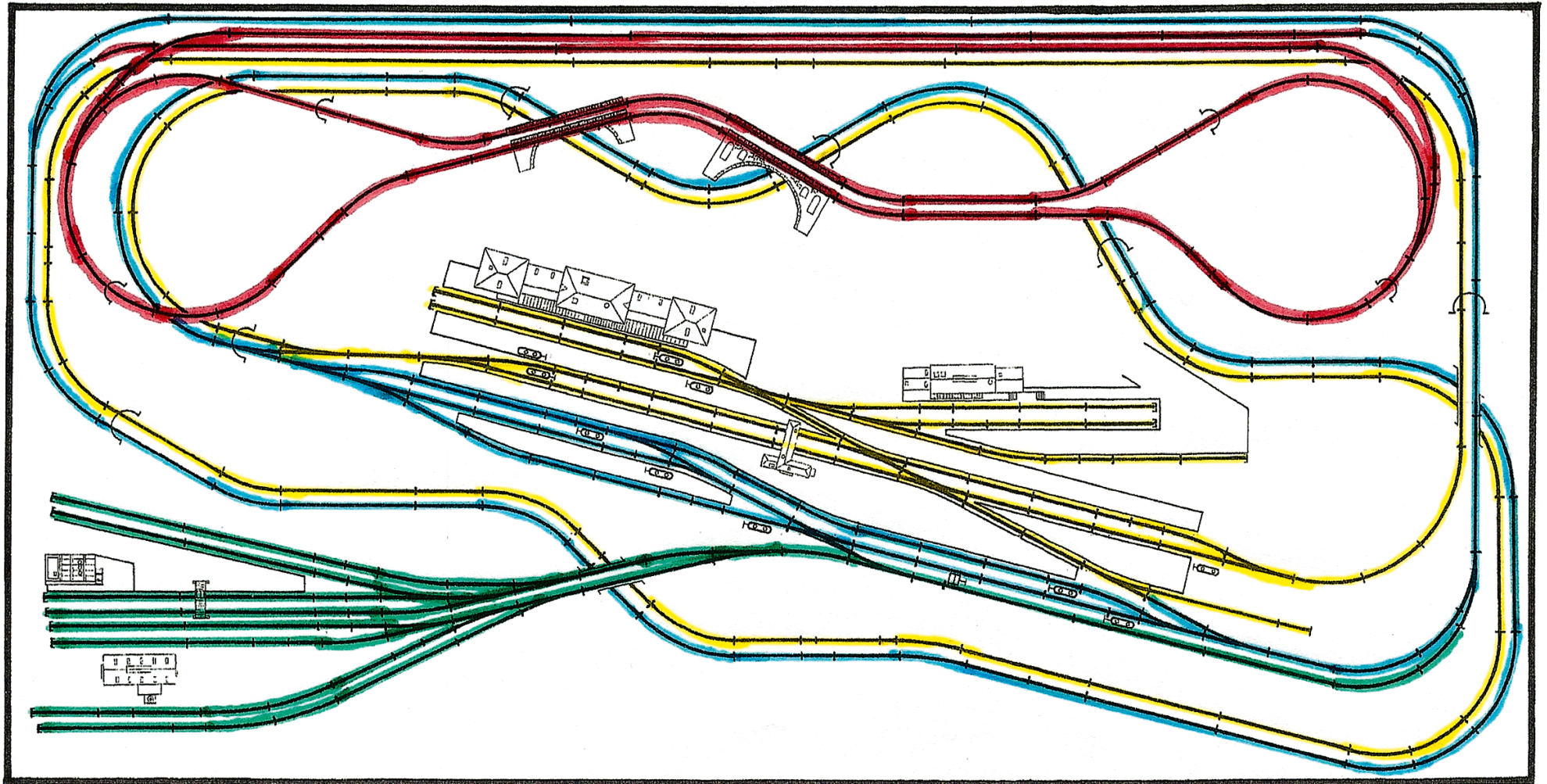
Vier verschiedene Stromkreise stehen für vier voneinander unabhängige Streckenabschnitte.
