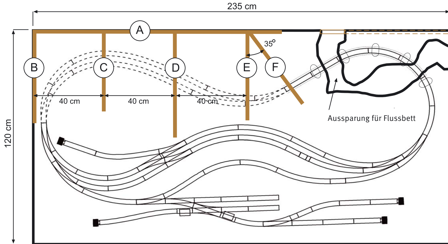
Spanten A bis F aus 16 mm dicken Stäbchenplatten als Unterbau für den Berg.
